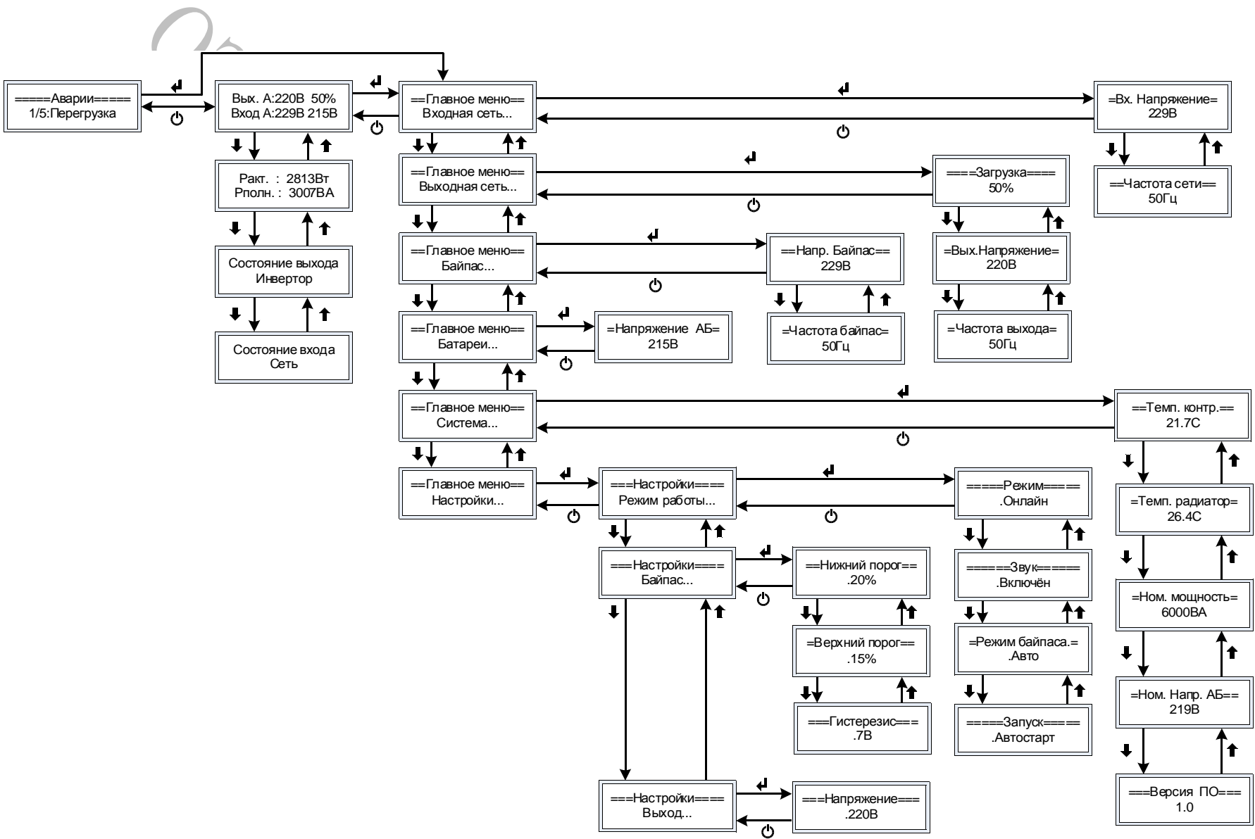
Рисунок 1.5 - Структура меню изделия
